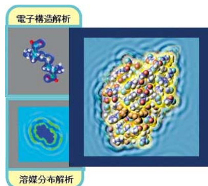
CSIを構成するNAREGIグリッドミドルウェアによる溶媒中のタンパク質連成計算
